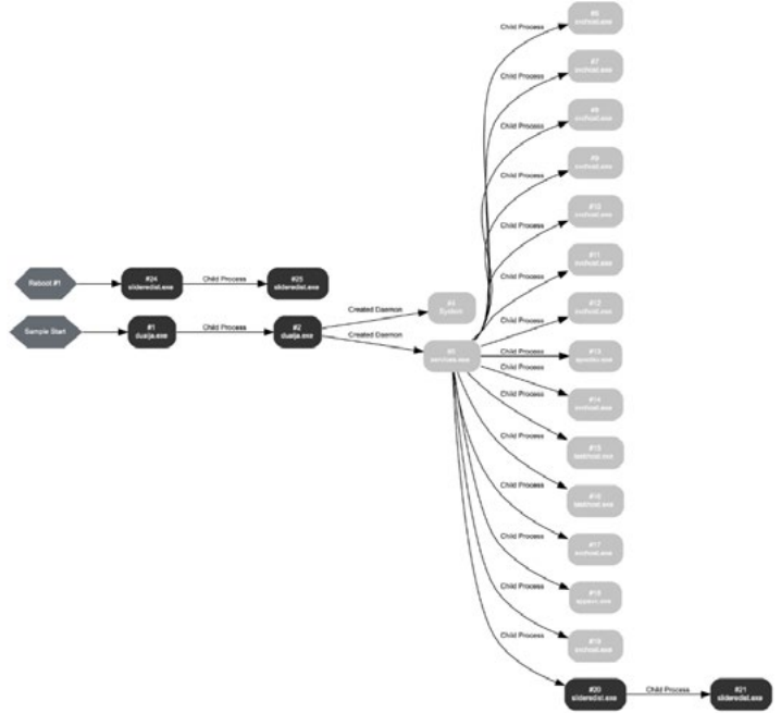
Şekil 64: İndirilen zararlı dosyanın süreç grafiği.
