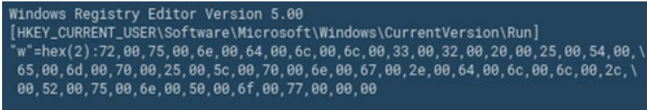
Şekil 35: Payload kodunu içeren kayıt defteri dosyası.
